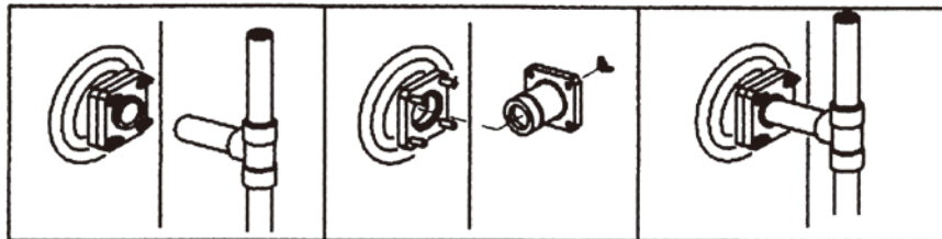
(1) 排水管をはずす
